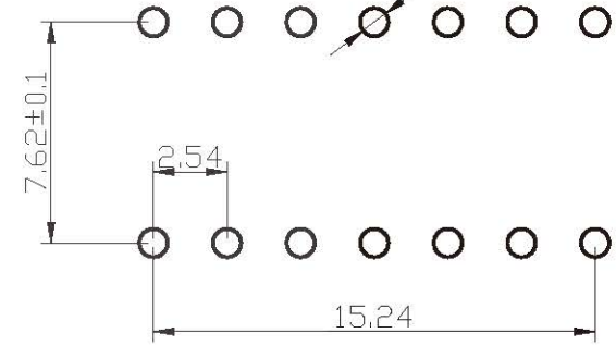
PCB开孔
