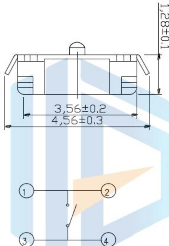
电路图
