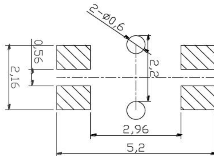
PCB. 焊接图
